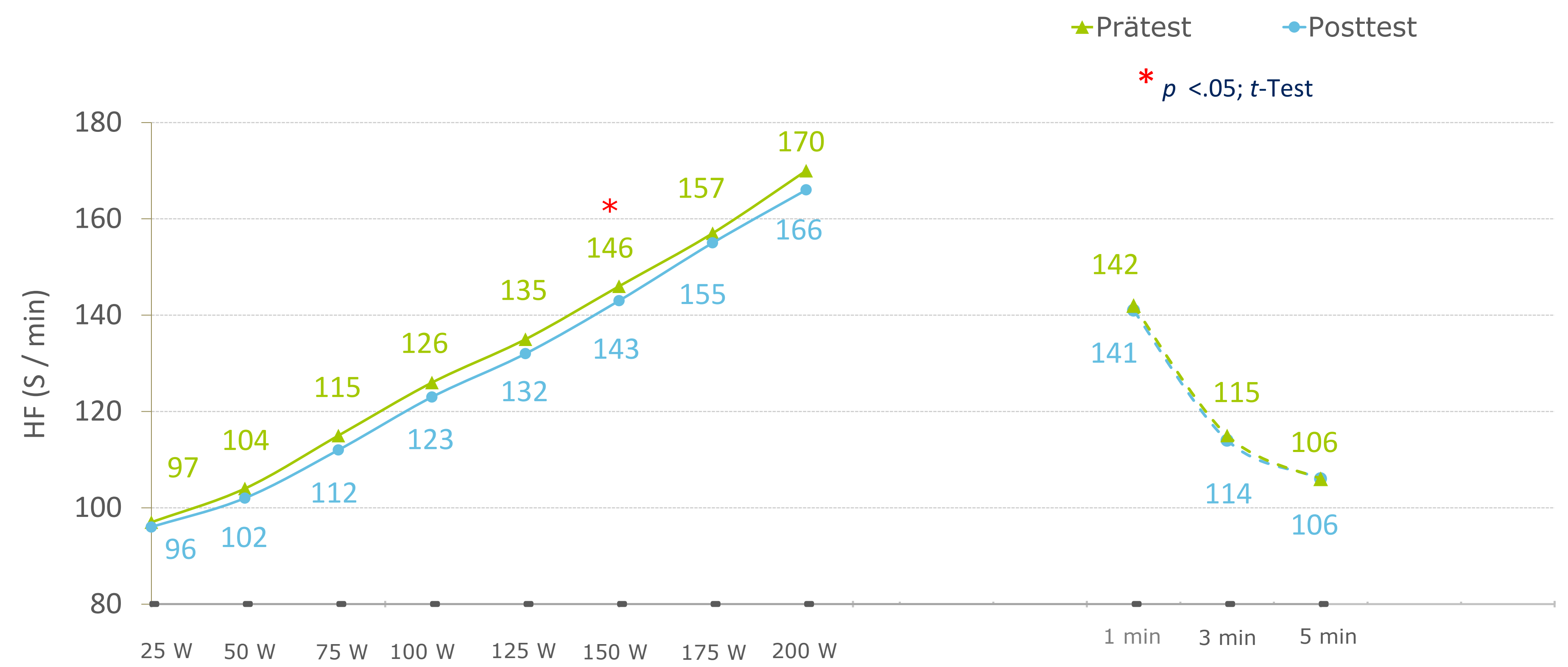
Leistung (Watt)
